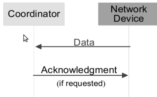
Fig. 4.12. Comunicació al coordinador PAN amb la balisa no habilitada
