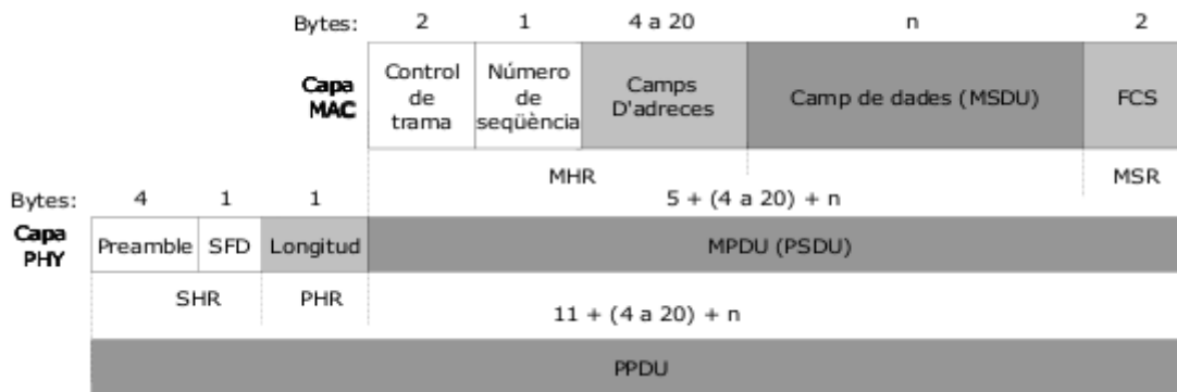
Fig. 4.8 Estructura de la trama de dades PHY+MAC
